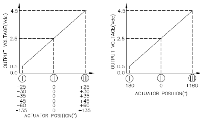
典型输出信号 Typical Output
